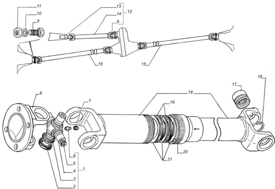
Рис. 11. Вали карданные трансмиссии
