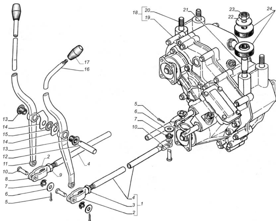
Рис. 7. Раздаточная коробка. Привод управления
