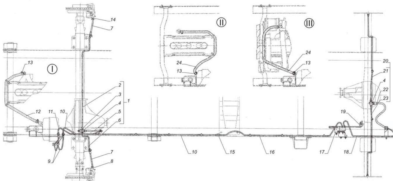
Рис. 15. Трубопроводы тормозной системы. I - автомобиля с двигателем 3М3-4063; II - с дв. 3М3-40522; III - с дв. ГАЗ-560
