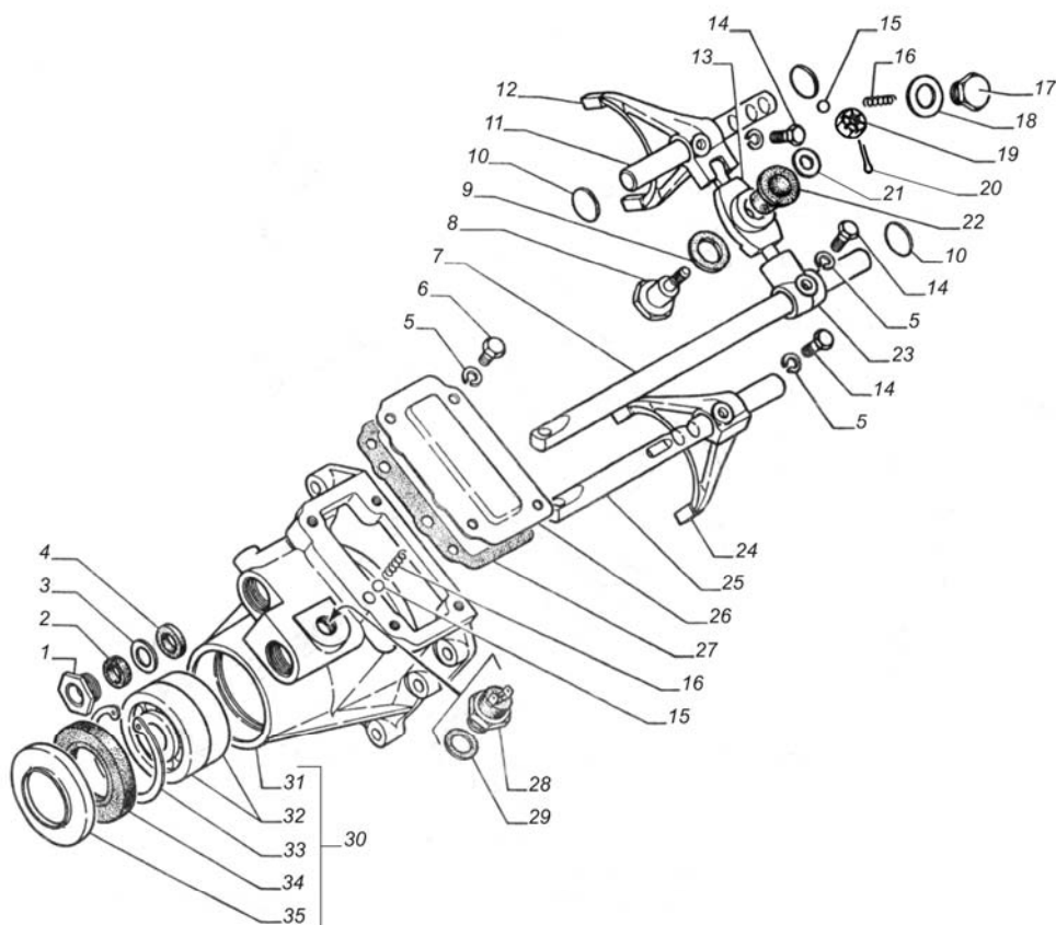
Рис. 9. Картер задний раздаточной коробки
