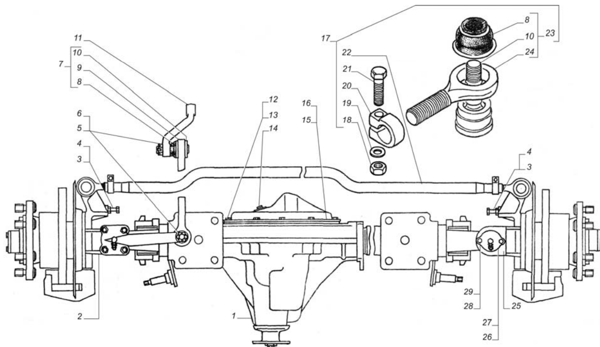
Рис. 3. Мост передний ведущий
