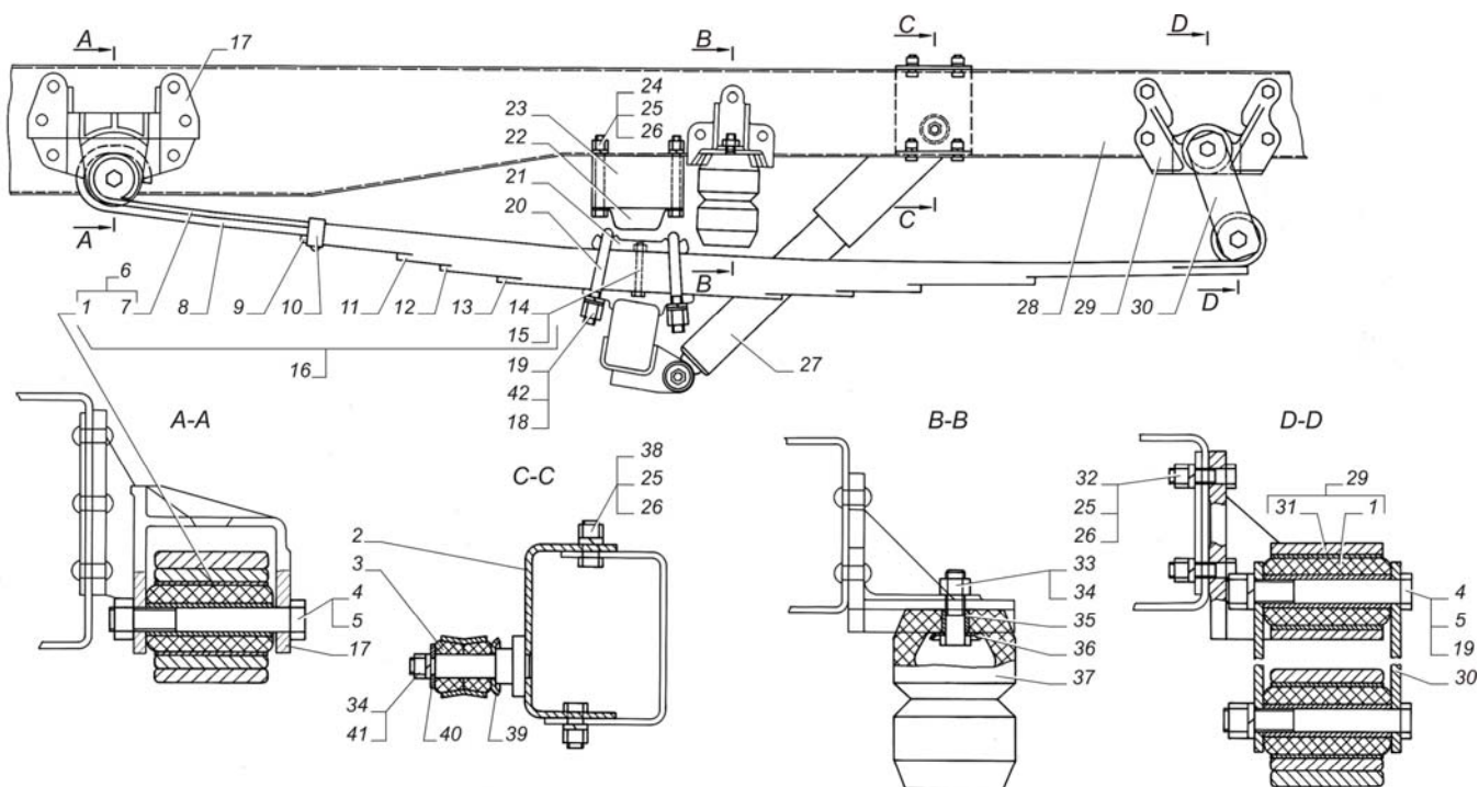
Рис. 13. Установка задней подвески
