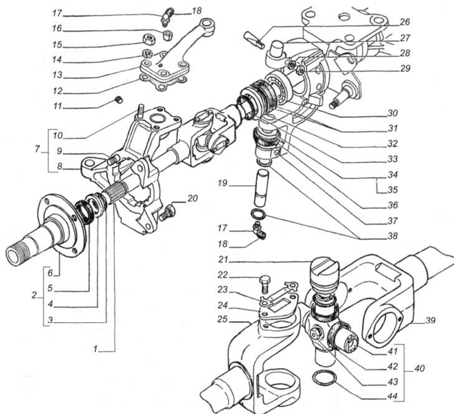
Рис. 5. Кулак поворотный переднего моста с шарниром
