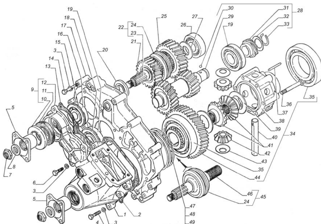
Рис. 8. Валы и шестерни раздаточной коробки
