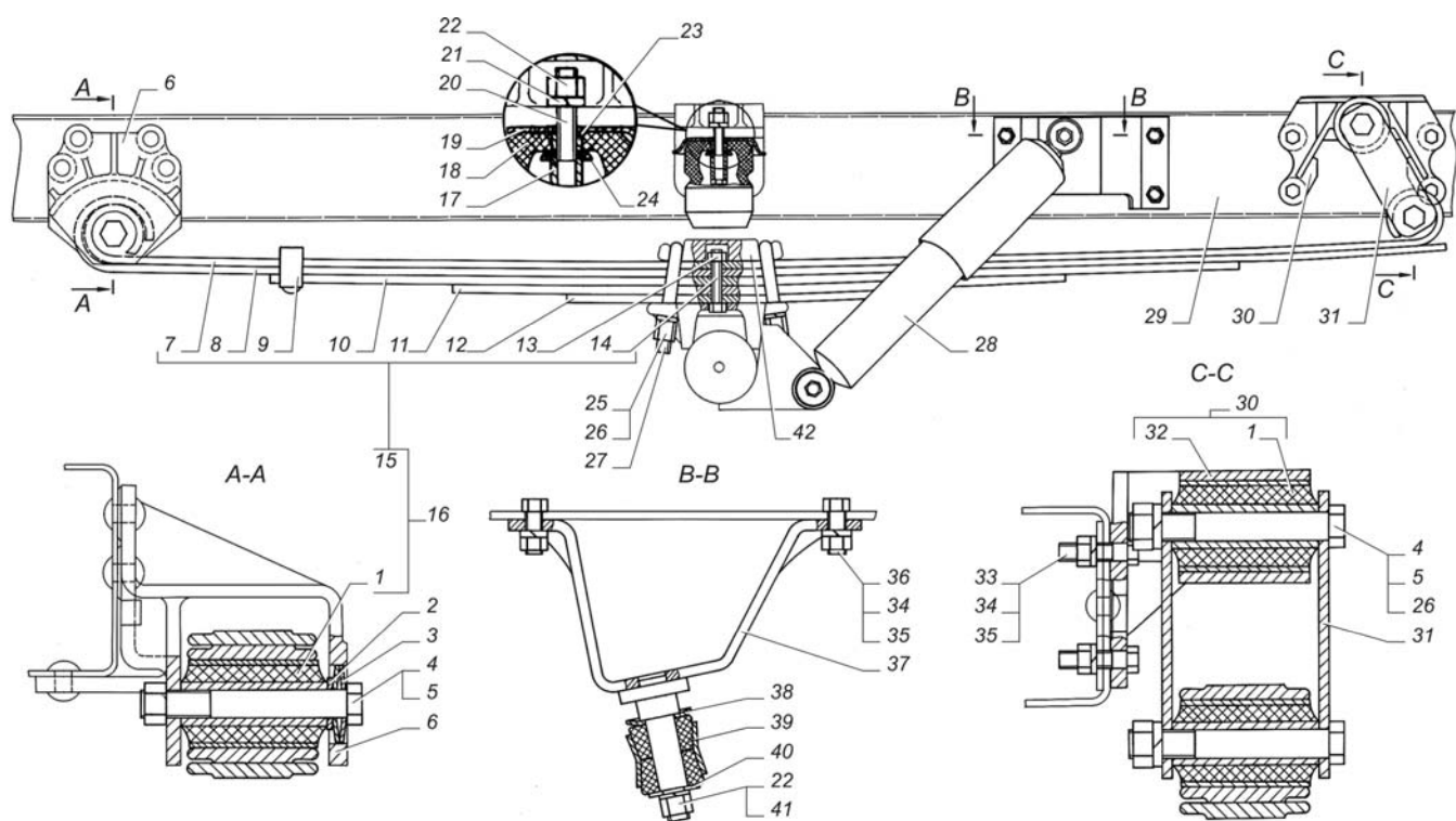
Рис. 12. Установка передней подвески
